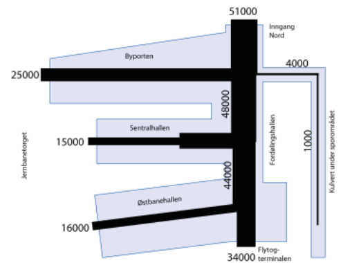
Figur 4 a og b Viser gangtrafikk gjennom Oslo S med adkomst fra Byporten, Sentralhallen, Østbanehallen, fra kulvert under sporene og inngang fra nord og sør. Figuren til venstre er trafikkprognose for yrkesdøgn (YDT) for 2028. Figuren over er trafikksituasjonen som ble registrert i 2005 (Kilde: Norsam 2007)
