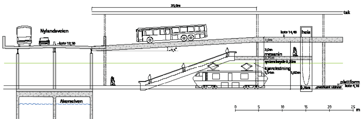
Figur 28 Snitt for terminal øst for Nylandsveien. Denne viser at lokket må heves for å få plass til mesalin mellom lokket og kjøreledningen for jernbane.
